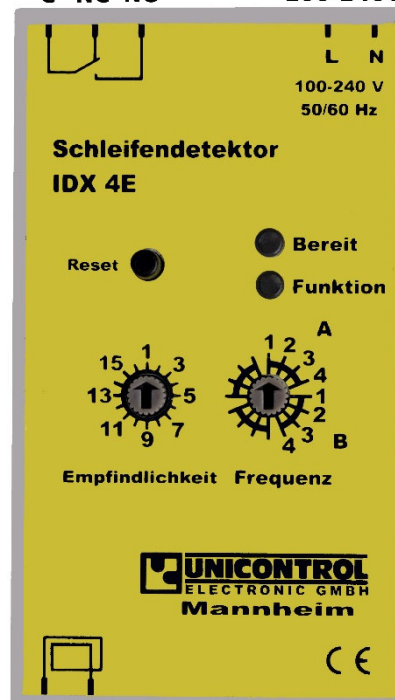
Induktionsschleife
